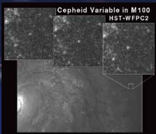
1：ハッブル望遠鏡が観測した銀河 (M100) 内の変光星 (Credit:NASA/STScI)
